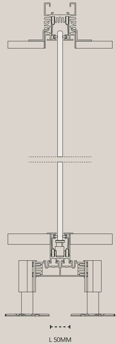
H1 PARETE VETRO SINGOLO | SINGLE-GLASS PARTITION WALL
